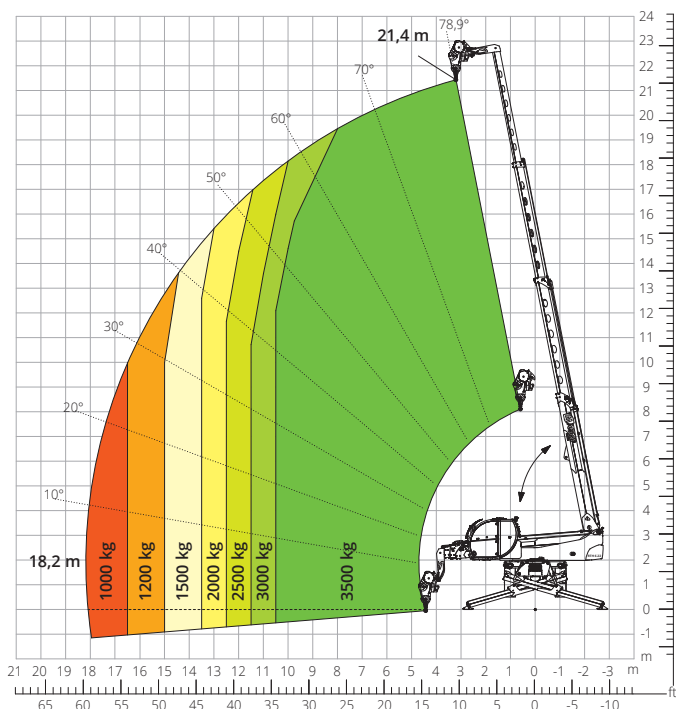
Lastdiagramm mit SEILWINDE 3.500 kg ATT - 02 - 002
