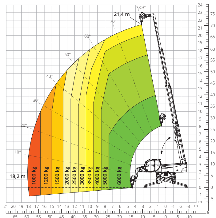
Lastdiagramm mit SEILWINDE 6.000 kg ATT - 02 - 004
