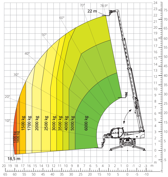
Lastdiagramm mit SEILWINDE 3.500 kg ATT - 02 - 002
