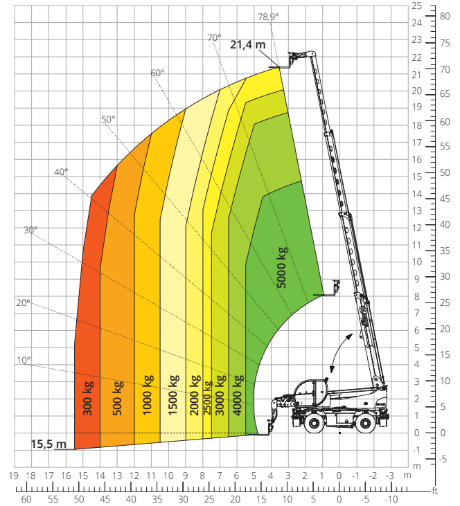
Lastdiagramm FRONTAL AUF REIFEN ATT-03-004
